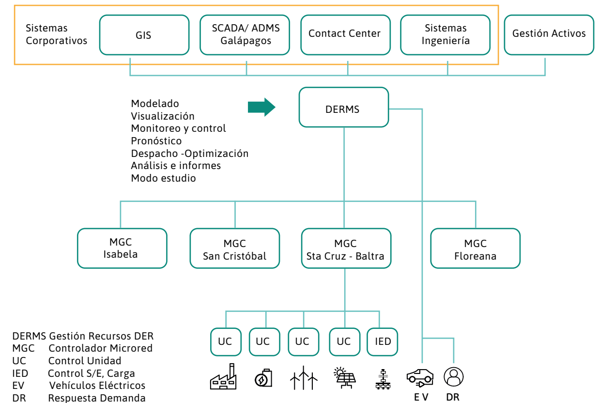
Figura 15 Esquema Conceptual de la Arquitectura del Sistema de Control 42
