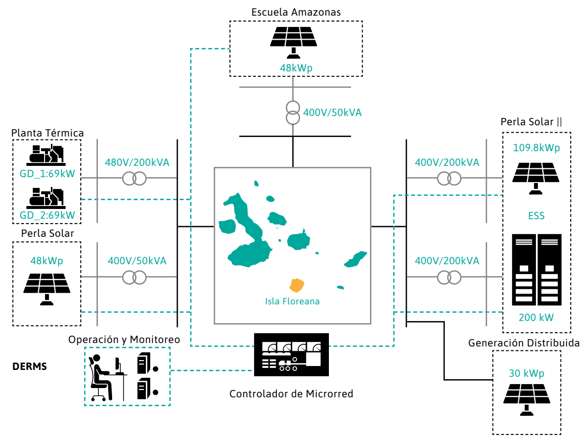
Figura 11 Diseño esquemático y constructivo para que la isla Floreana alcance el 100 % de renovable
