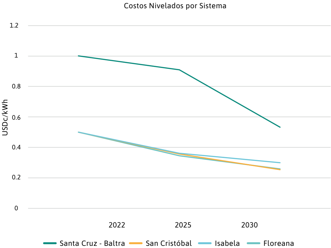
Figura 9 Costos Nivelados de Energía 2022 - 2030
