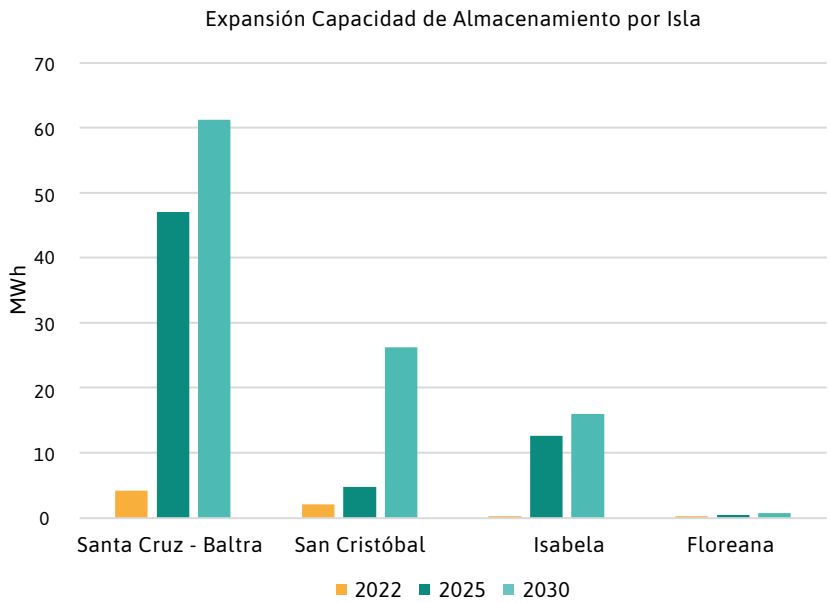
Figura 12 Expansión Capacidad de Almacenamiento por Isla
